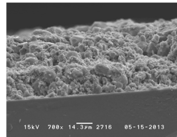
フォスセラ断面
