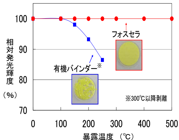
耐熱試験結果
